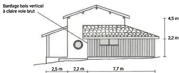
FAÇADE EST
