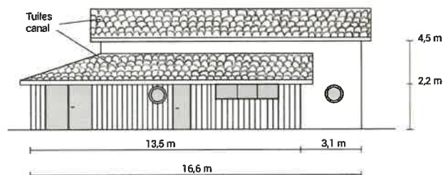
FAÇADE NORD
