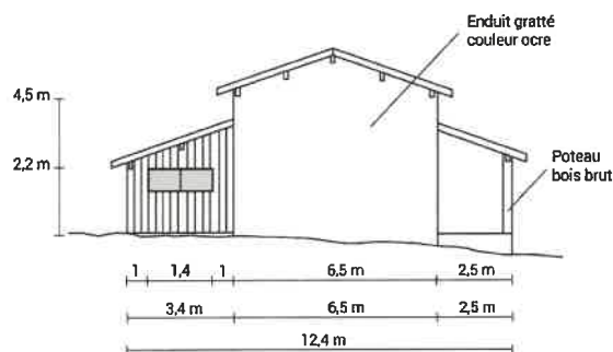
FAÇADE OUEST
