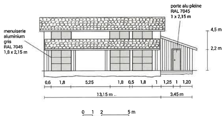
FAÇADE SUD
